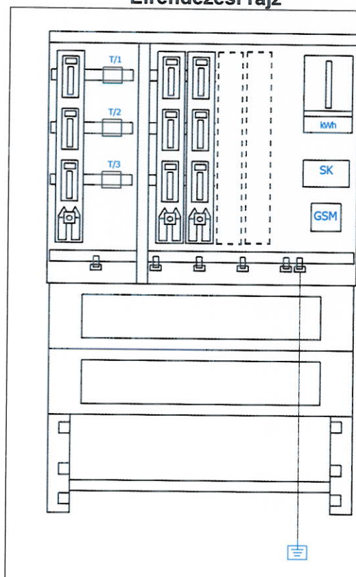
Elrendezési rajz
