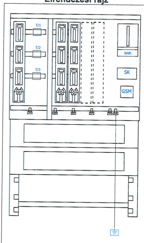
Elrendezési rajz
