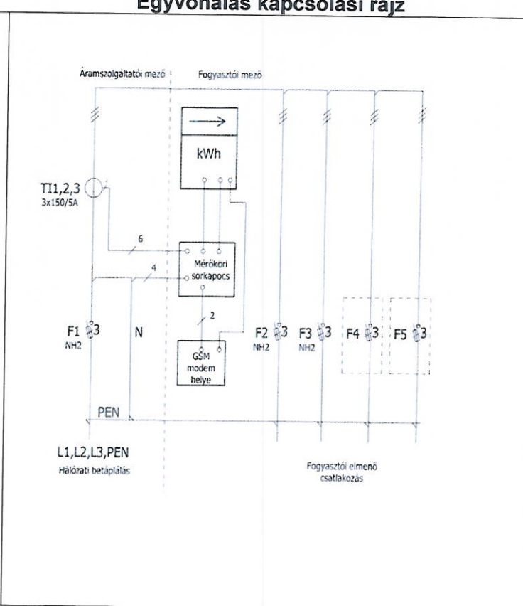
Egyvonalas kapcsolási rajz
