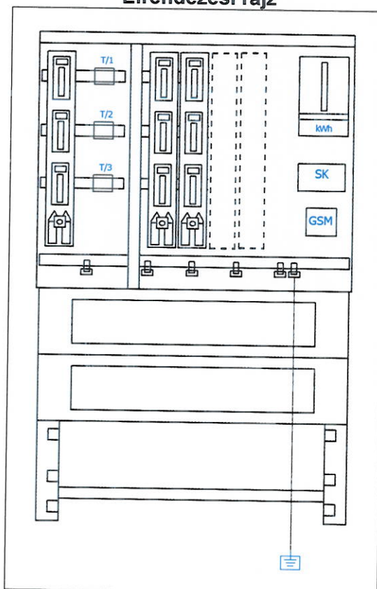
Elrendezési rajz
