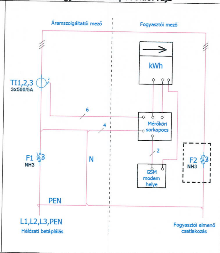
Egyvonalas kapcsolási rajz
