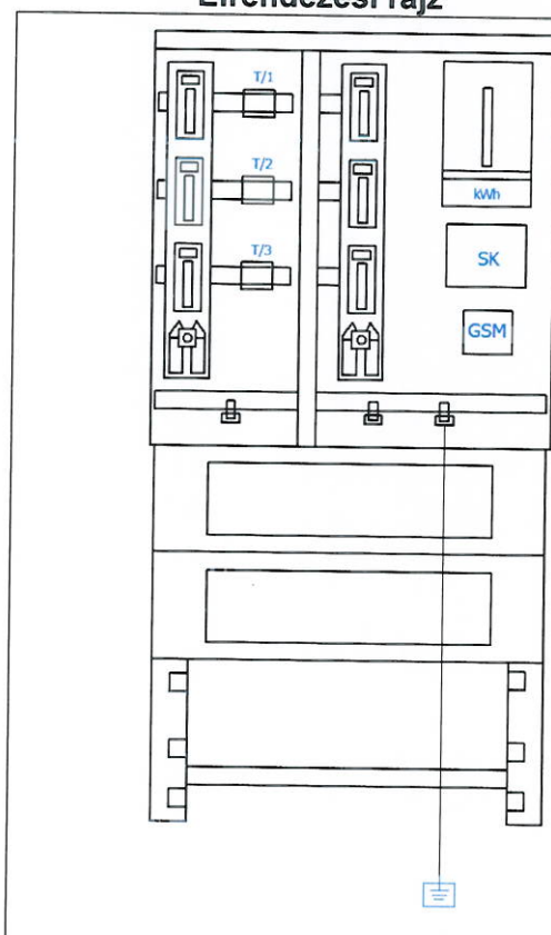
Elrendezési rajz
