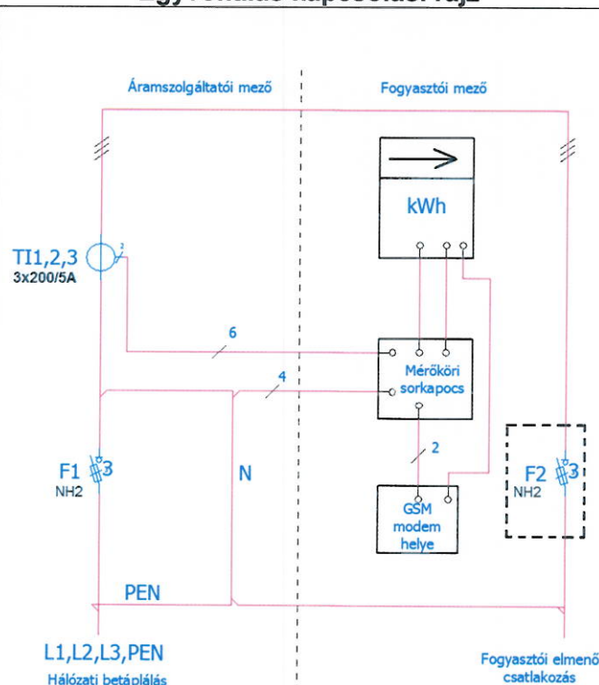
Egyvonalas kapcsolási rajz
