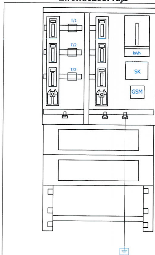
Elrendezési rajz
