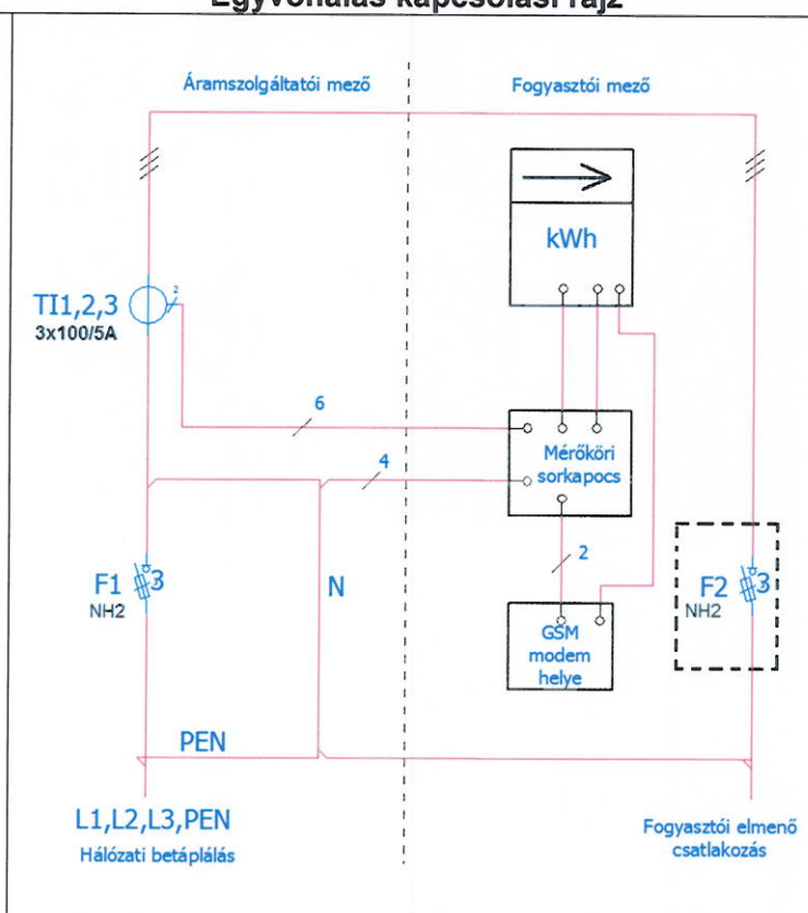
Egyvonalas kapcsolási rajz
