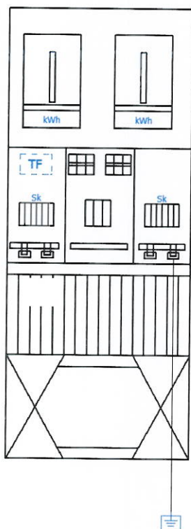
Elrendezési rajz
