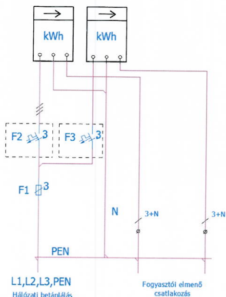
Egyvonalas kapcsolási rajz
