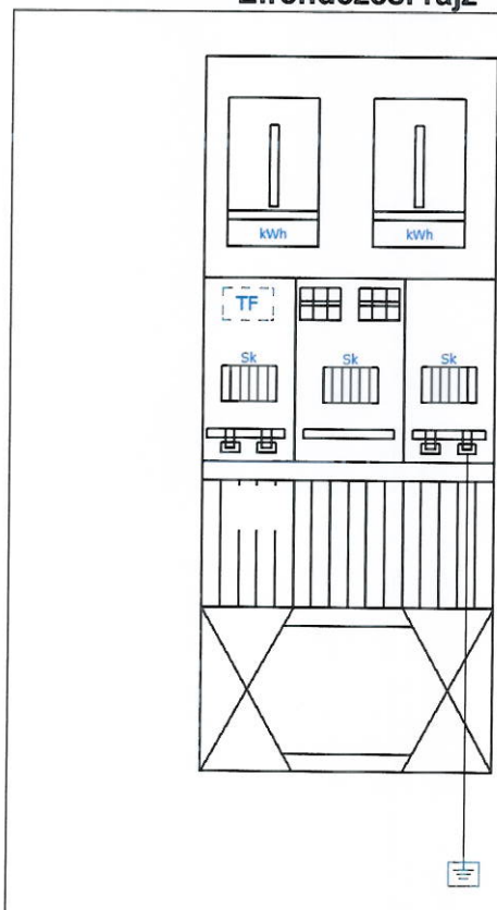
Elrendezési rajz
