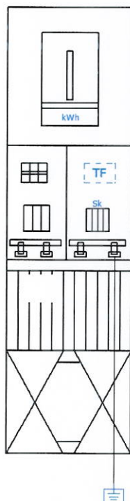
Elrendezési rajz
