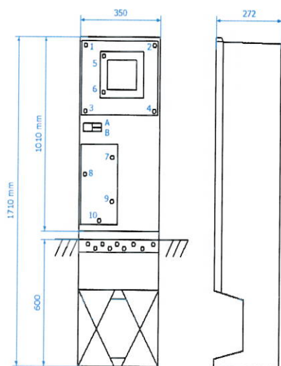
Méretezett körvonalrajz, plombálási helyek
