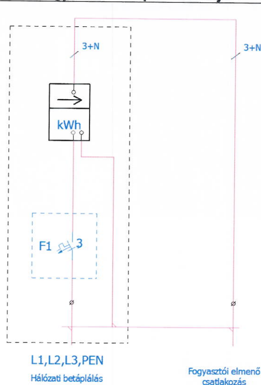
Egyvonalas kapcsolási rajz
